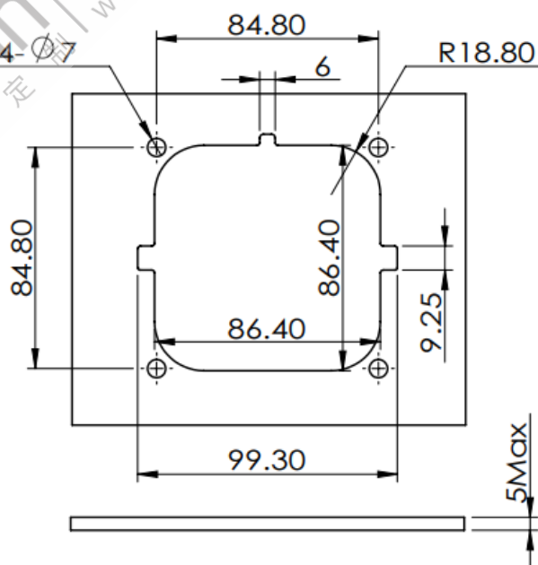
后安装方式尺寸参数
