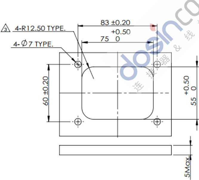
前安装方式尺寸参数
