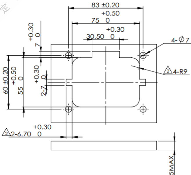
后安装方式尺寸参数
